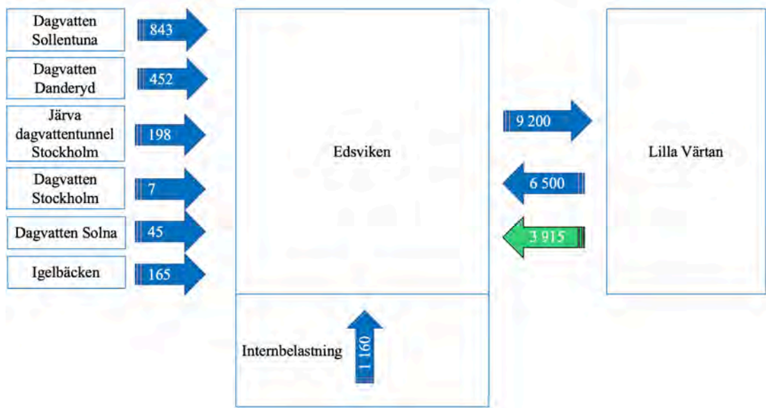
Figur 13. Boxmodell för fosfortransport (kg/år) från inflöden till Edsviken och utflöde från Edsviken till Lilla Värtan, där blå pilar anger den aktuella statusen och de gröna pilarna är belastningen till och från Lilla Värtan när den har god status.
