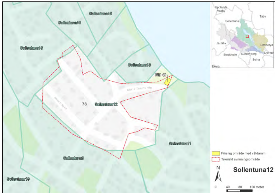
Figur 5. Delavrinningsområde 12 med förslag till placering av ny våtdamm.
