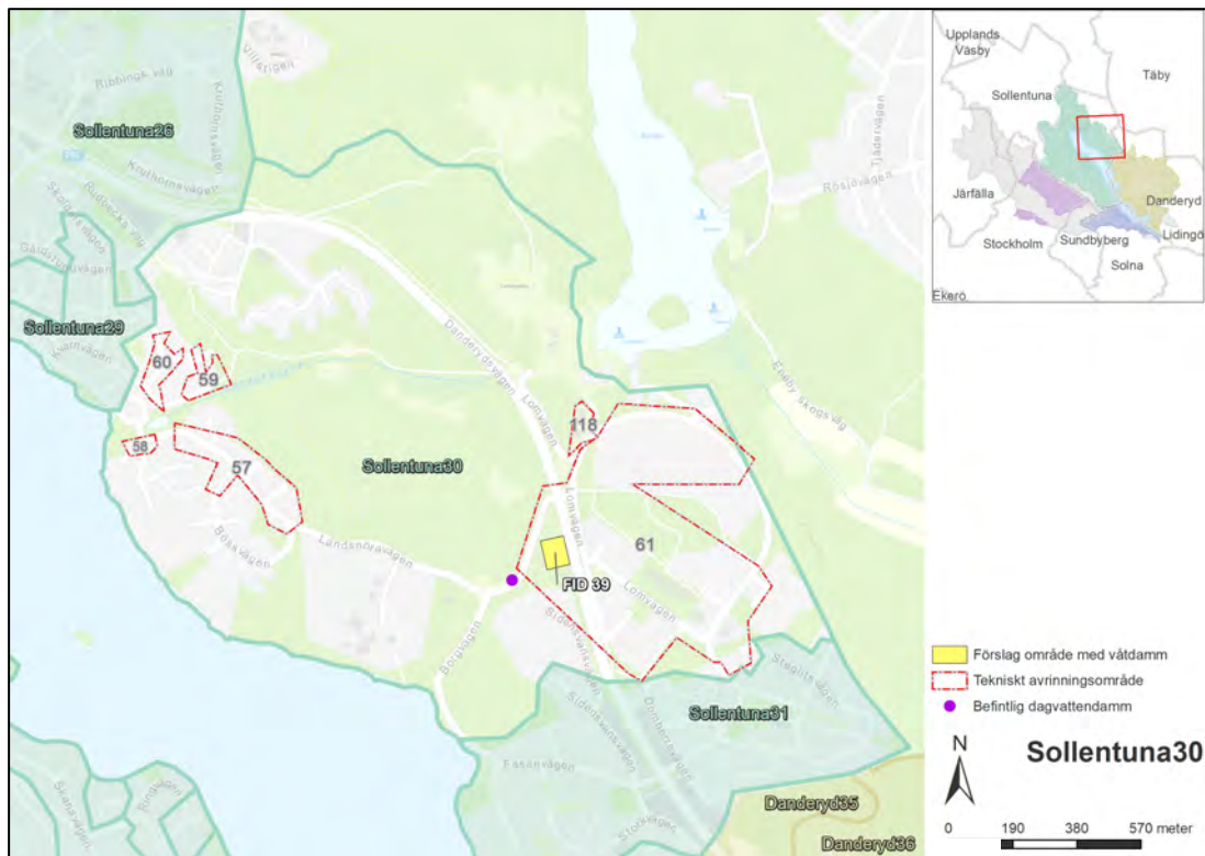
Figur 15. Delavrinningsområde 30 med förslag till placering av våtdamm.
